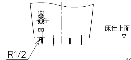
正面図 床給水仕様の場合
